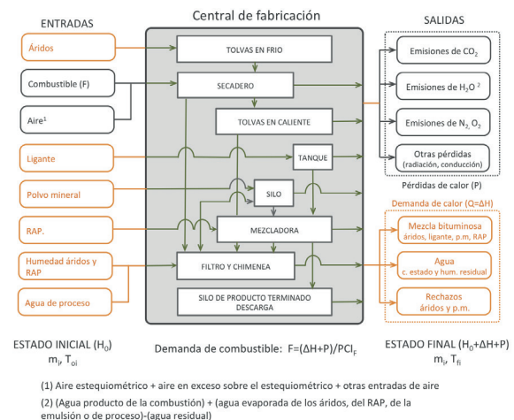
Figura 4: Diagrama de flujo para demanda de combustible.
