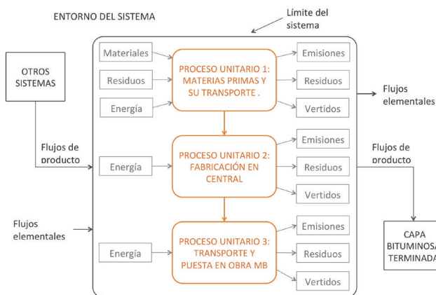
Figura 2: Diagrama de flujo general para la fabricación y puesta en obra de mezcla bituminosa en caliente según ECCO2.
