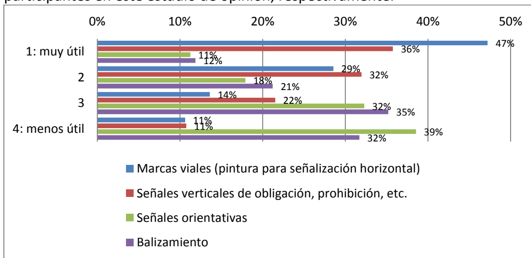
Elementos de mayor utilidad en la vía (1: más útil; 4: menos útil)
